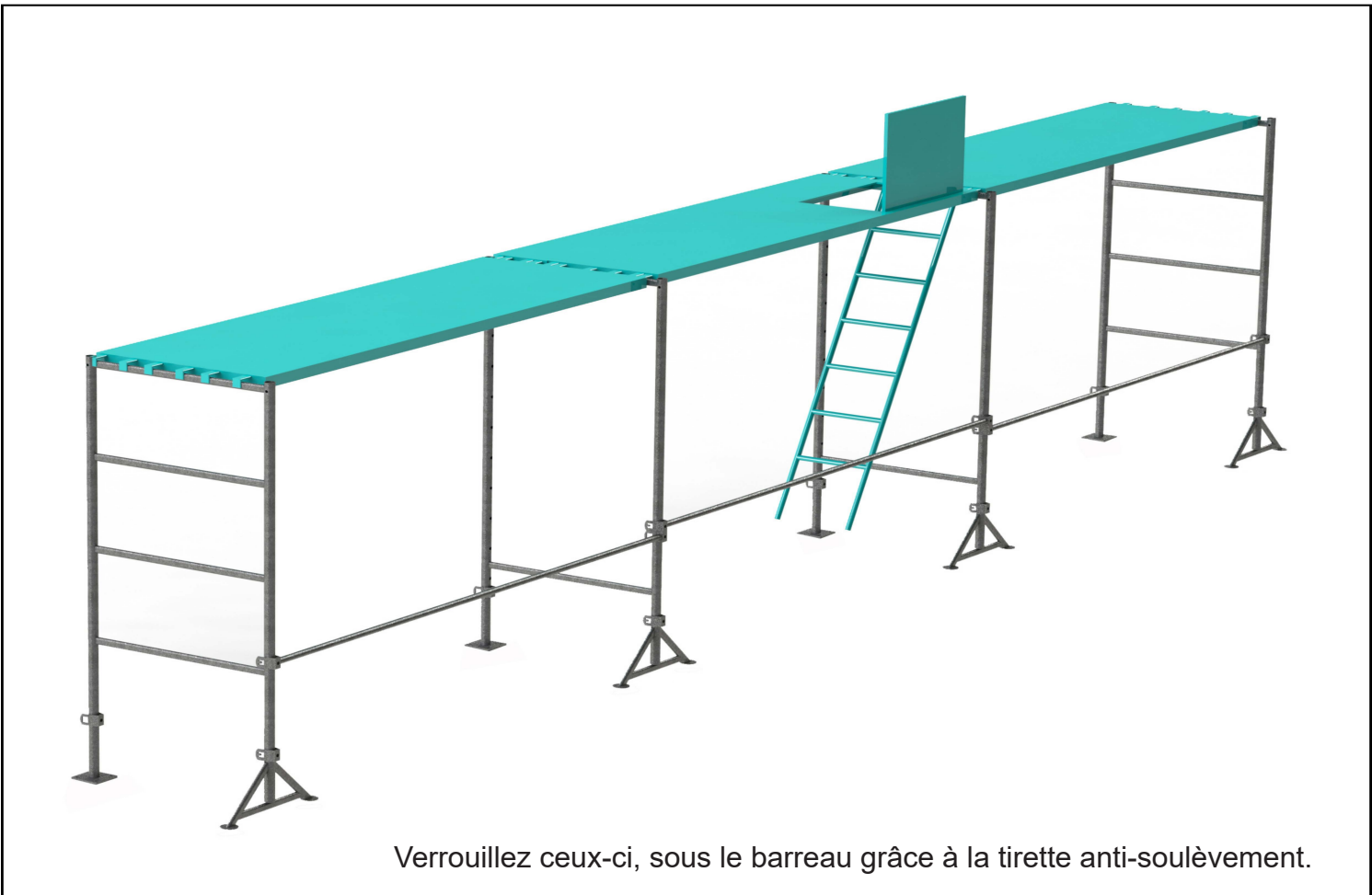
Configuration 2 : À 2 m du sol, installez l'échelle d'accès, sous le plancher trappe
