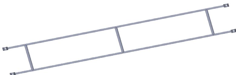
GARDE-CORPS FIXE Longueur : 3 m Réf : ES49010
